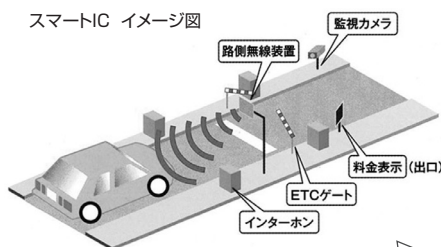
スマートIC イメージ図
